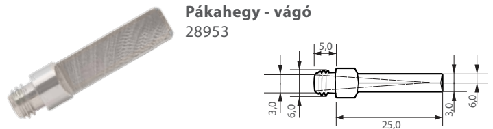
Pákahegy - vágó
